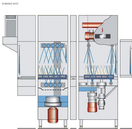
图解机器截面
